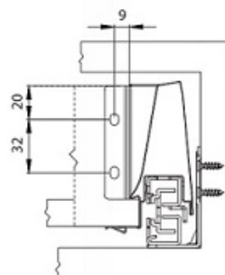
Wymiary montażowe ścianki tylnej
