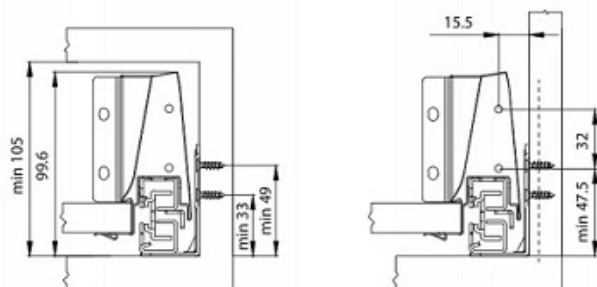
Wymiary montażowe szuflady i korpusu
