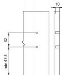
Wymiary montażowe frontu
